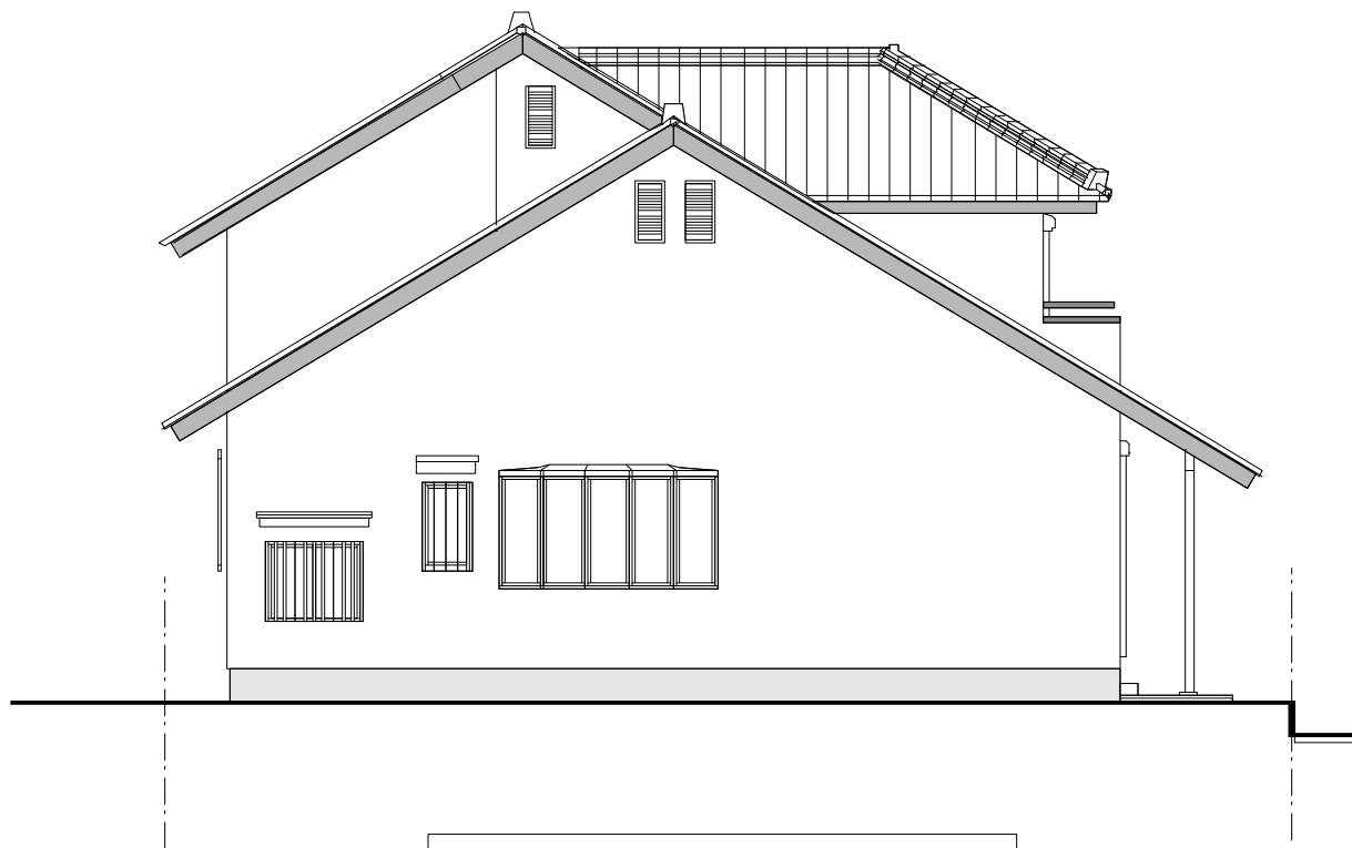
西側 立面図 1/100
