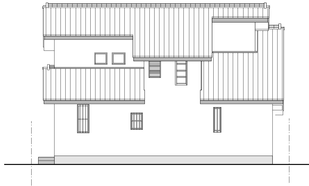
北側 立面図 1/100
