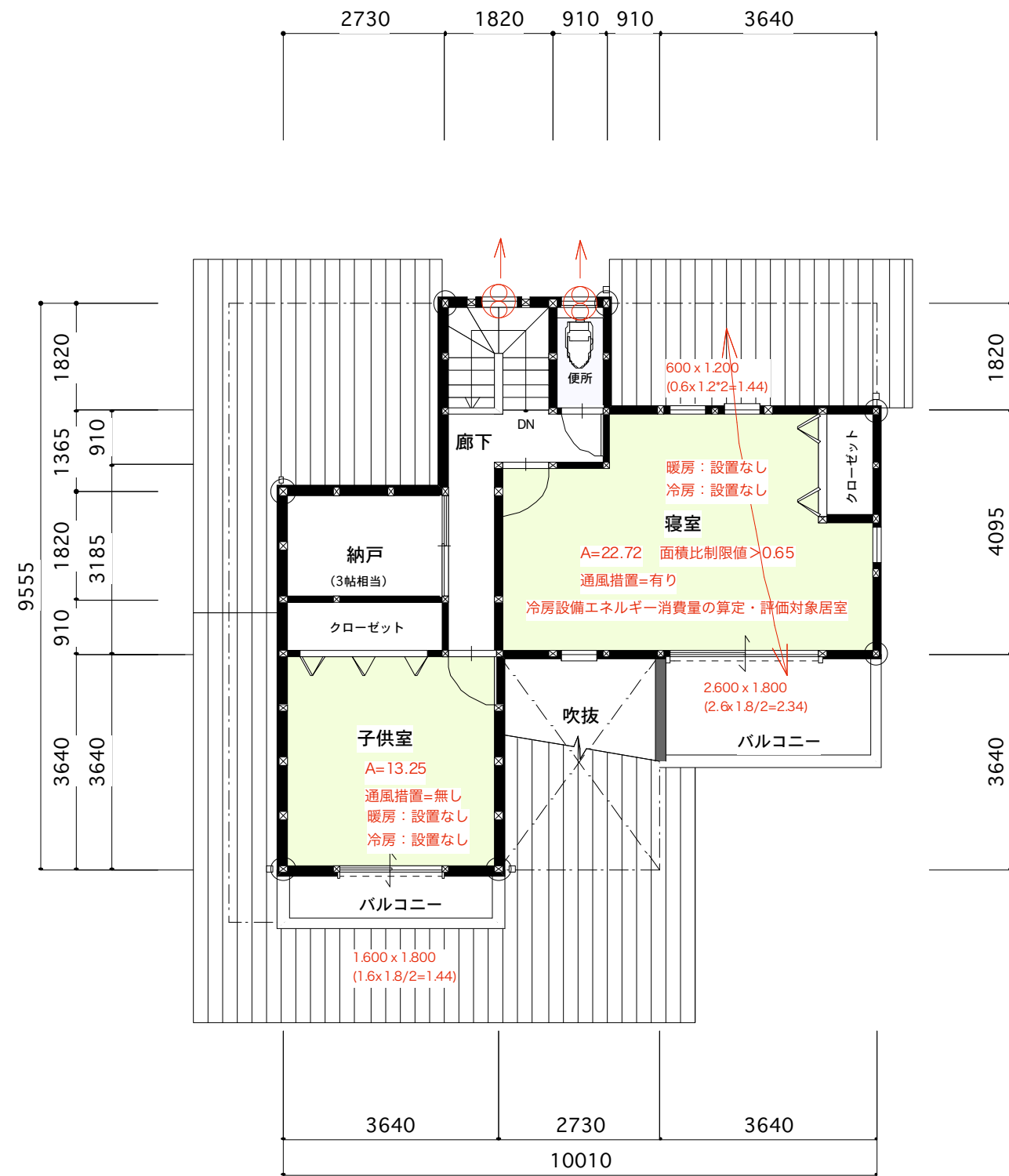
2階平面図 1/100
